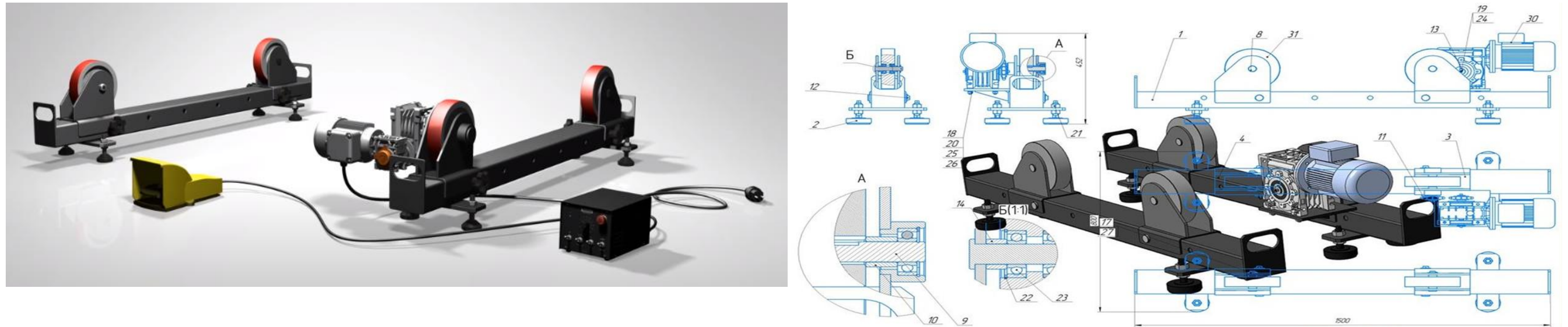
Рис.1 Роликовый вращатель с приводом вращения
