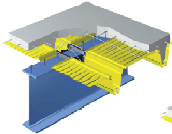
стальная балка
