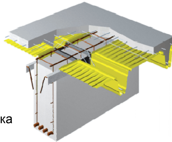
железобетонная балка - готовый элемент
