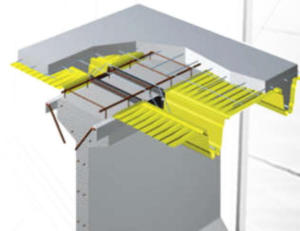
железобетонная балка - готовый элемент
