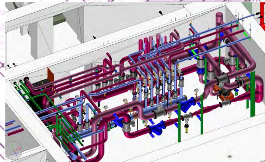
ВМ-модель. Индивидуальный тепловой пункт
