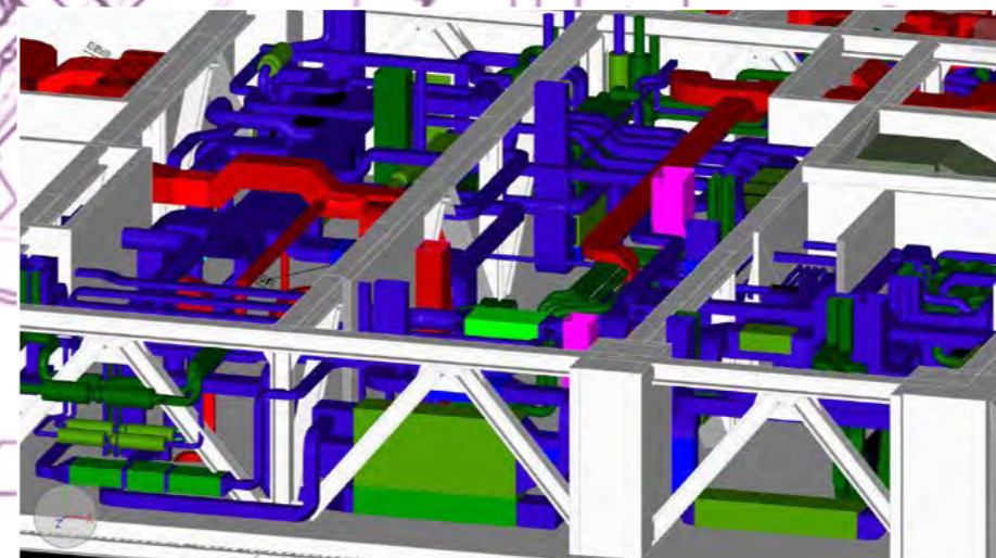
ВМ-модель. Фрагмент технического этажа
